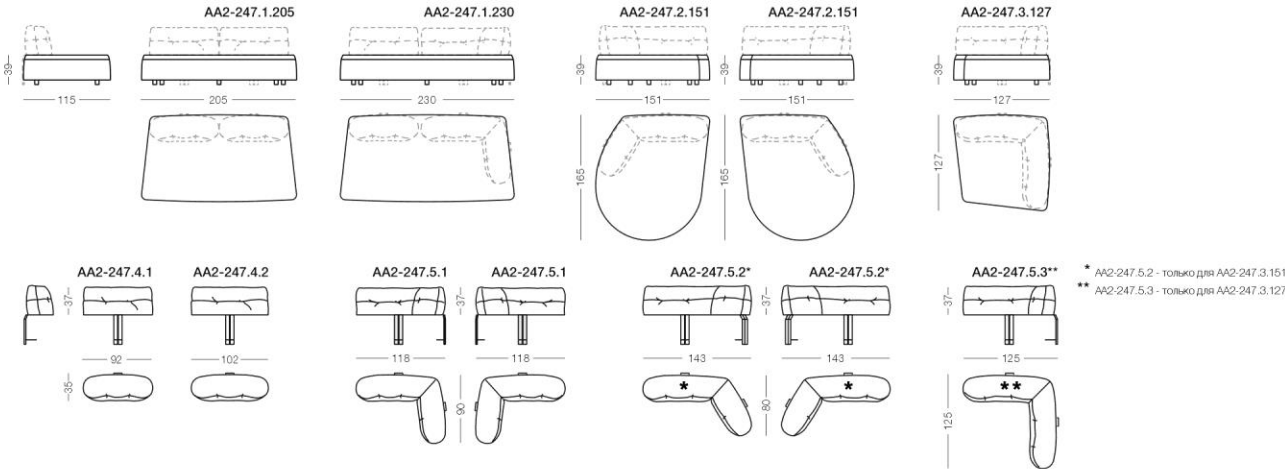
Варианты компоновки модулей
